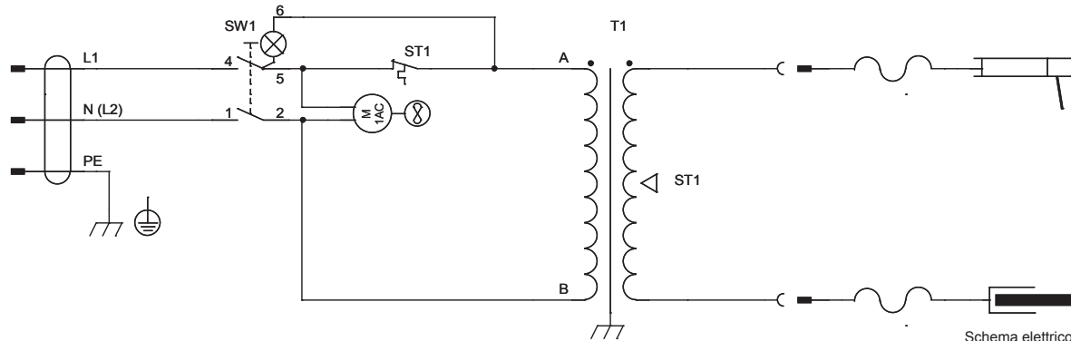
Schema elettrico N. Schéma électrique N. Diagram N. Schaltplan N. Esquema de conexiones N.
